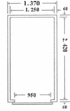
AS/300 SENZA PAVIMENTO CARRELLO
