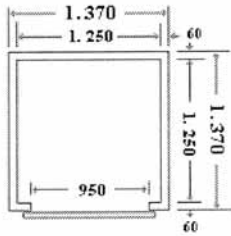
AS/150 PAVIMENTO CARRELLO E PEDANA
