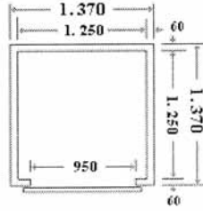
AS/150 SENZA PAVIMENTO CARRELLO
