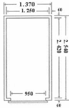
AS/300 PAVIMENTO CARRELLO E PEDANA
