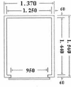
AS/200 SENZA PAVIMENTO CARRELLO
