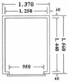
AS/200 PAVIMENTO CARRELLO E PEDANA
