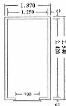
AS/300 PAVIMENTO ASTE PORTA SALUMI
